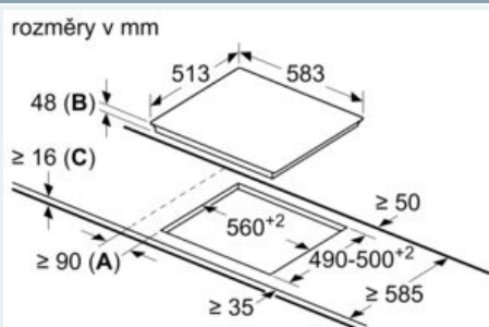
Rozměrové výkresy
