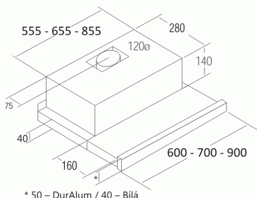
Rozměry v mm
